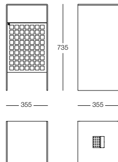
steel plate litter bin 35L corbeille en acier 35L papeleira em chapa 35L
