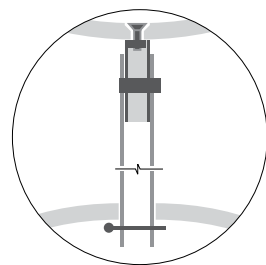
outdoor benches water drainage scheme système de drainage d'eau pour bancs d'extérieur escoamento de águas para bancos de exterior
