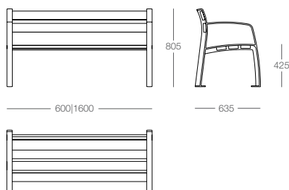
bench with backrest banc avec dossier banco com costas
