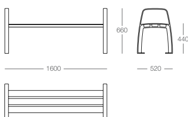
bench without backrest and with armrest banc sans dossier et avec support de bras banco sem costas e com apoio de braços
