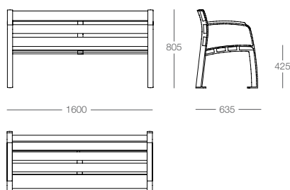
Elegance Confort bench with backrest banc avec dossier Elegance Confort banco com costas Elegance Confort
